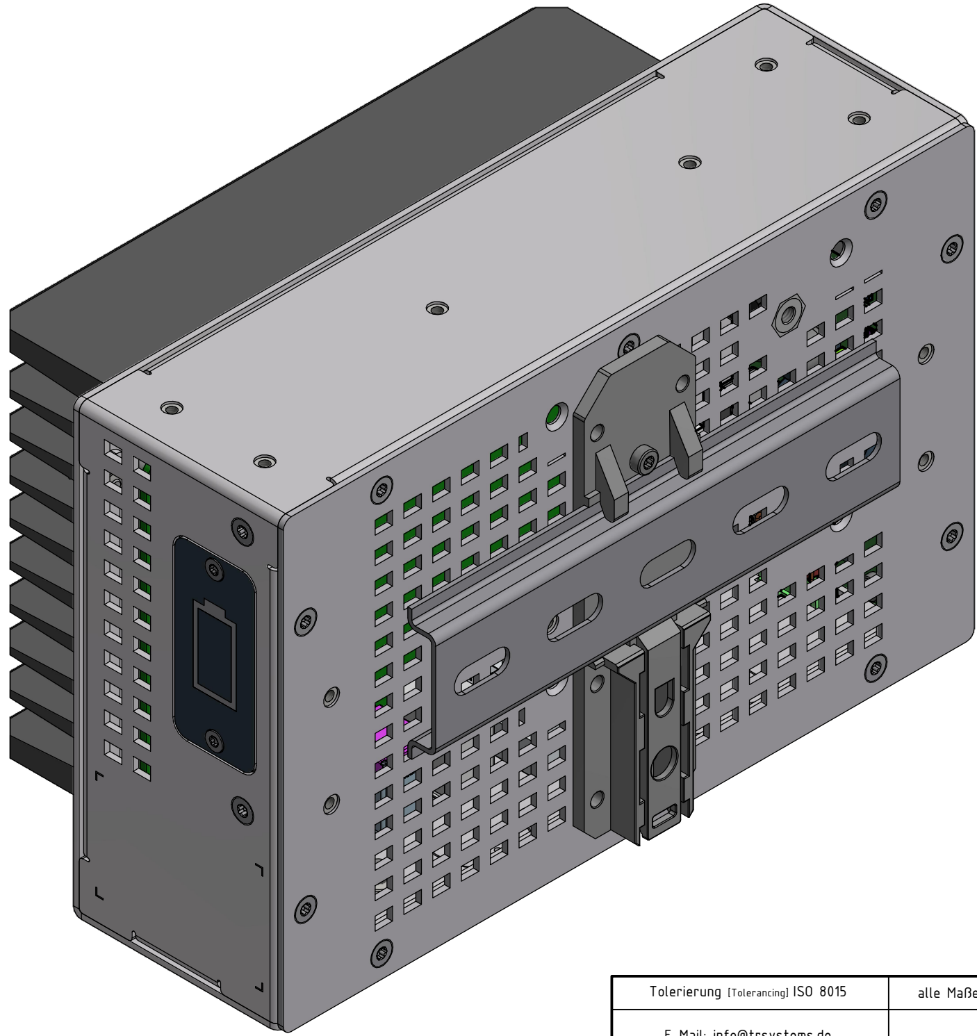
Montageart 2
